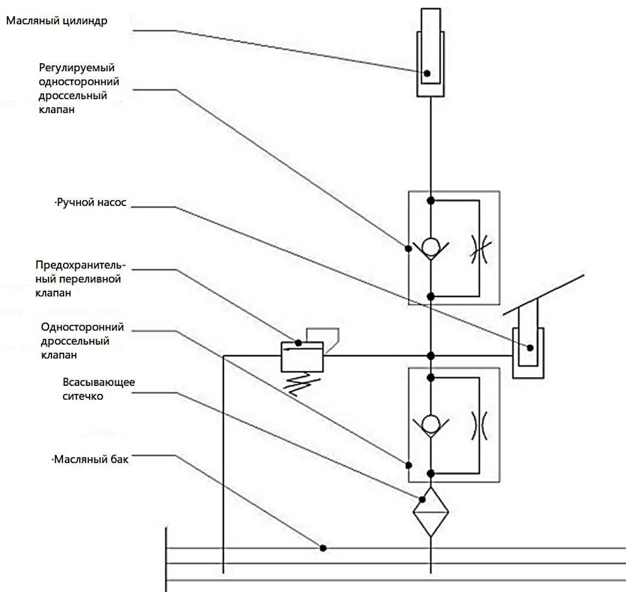
Рис.3 - Схема гидравлической системы
